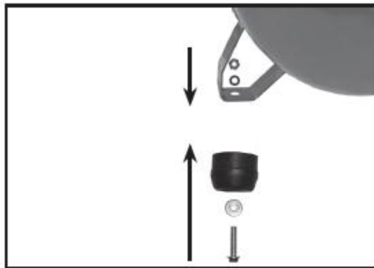
Рисунок. Установка амортизаторов на компрессор.
